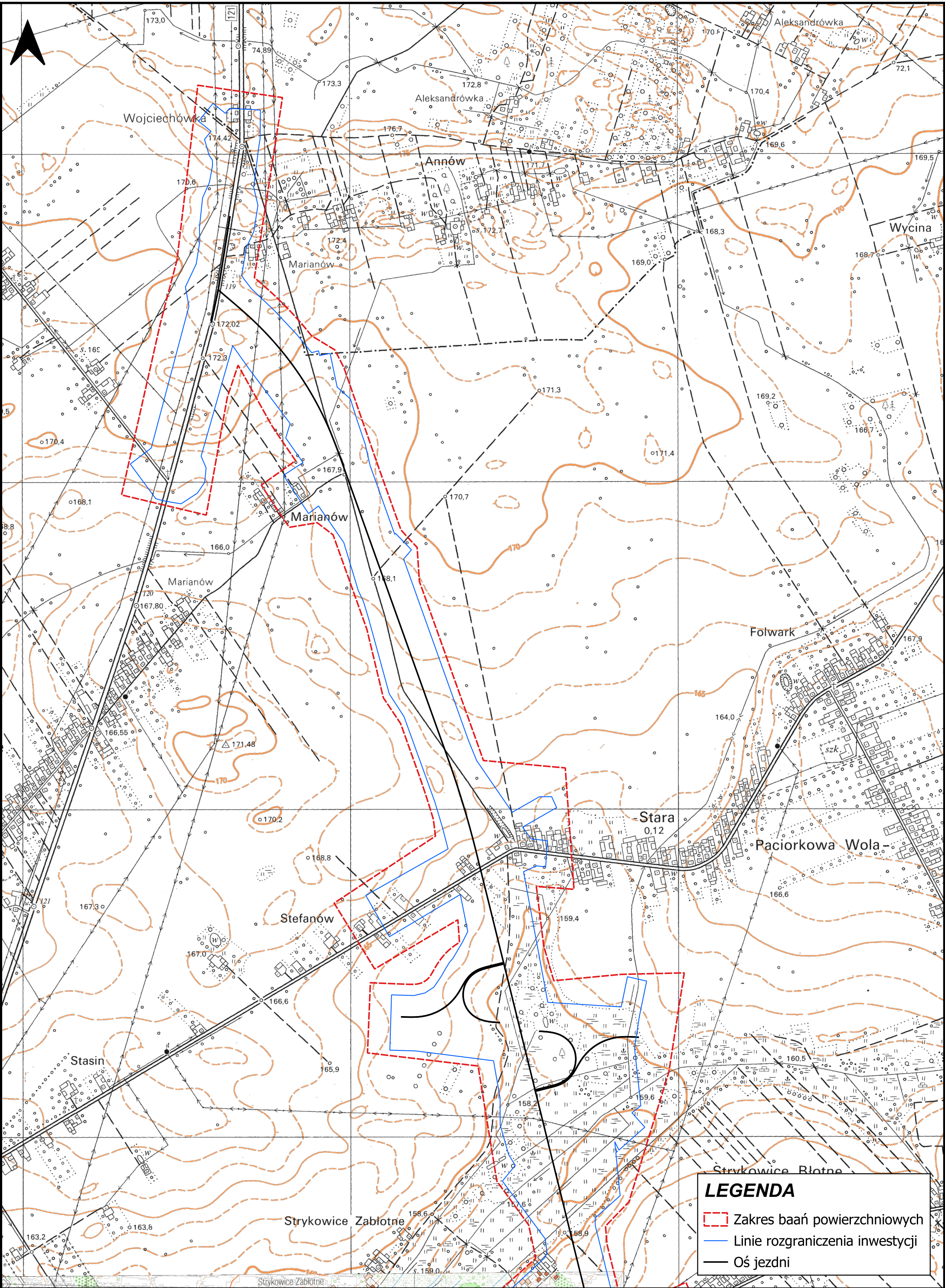
Wykonanie badań powierzchniowych dla zadania: "Budowa Obwodnicy Zwolenia w ciągu drogi krajowej nr 79" 0 250 500 750 1 000 m
