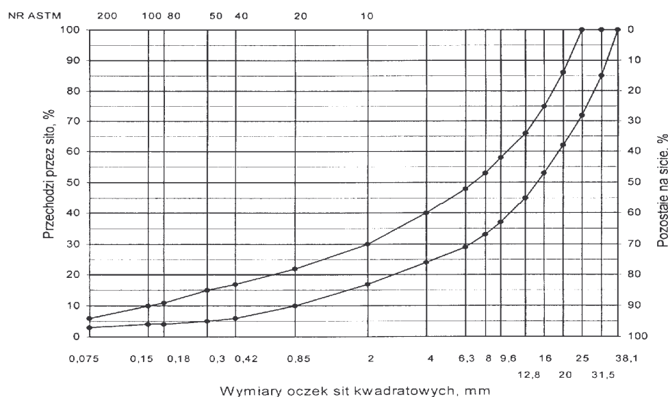
Rys. 1. Krzywe graniczne uziarnienia mieszanki mineralnej BA od 0 do 25 mm podbudowy nawierzchni drogi o obciążeniu ruchem KR 3 i KR 6.
