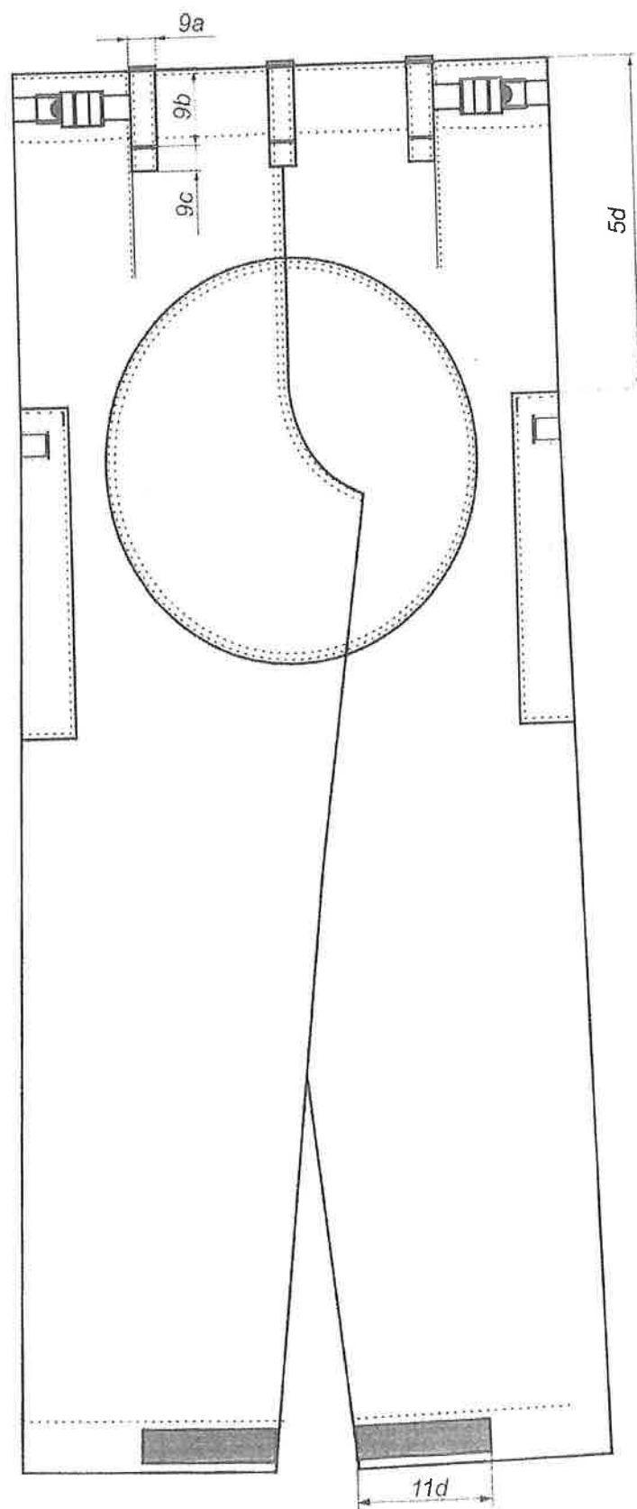
Rysunek 7-Tył spodni
