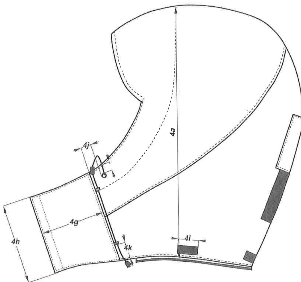
Rysunek 4 - Kurtka - góra tyłu
