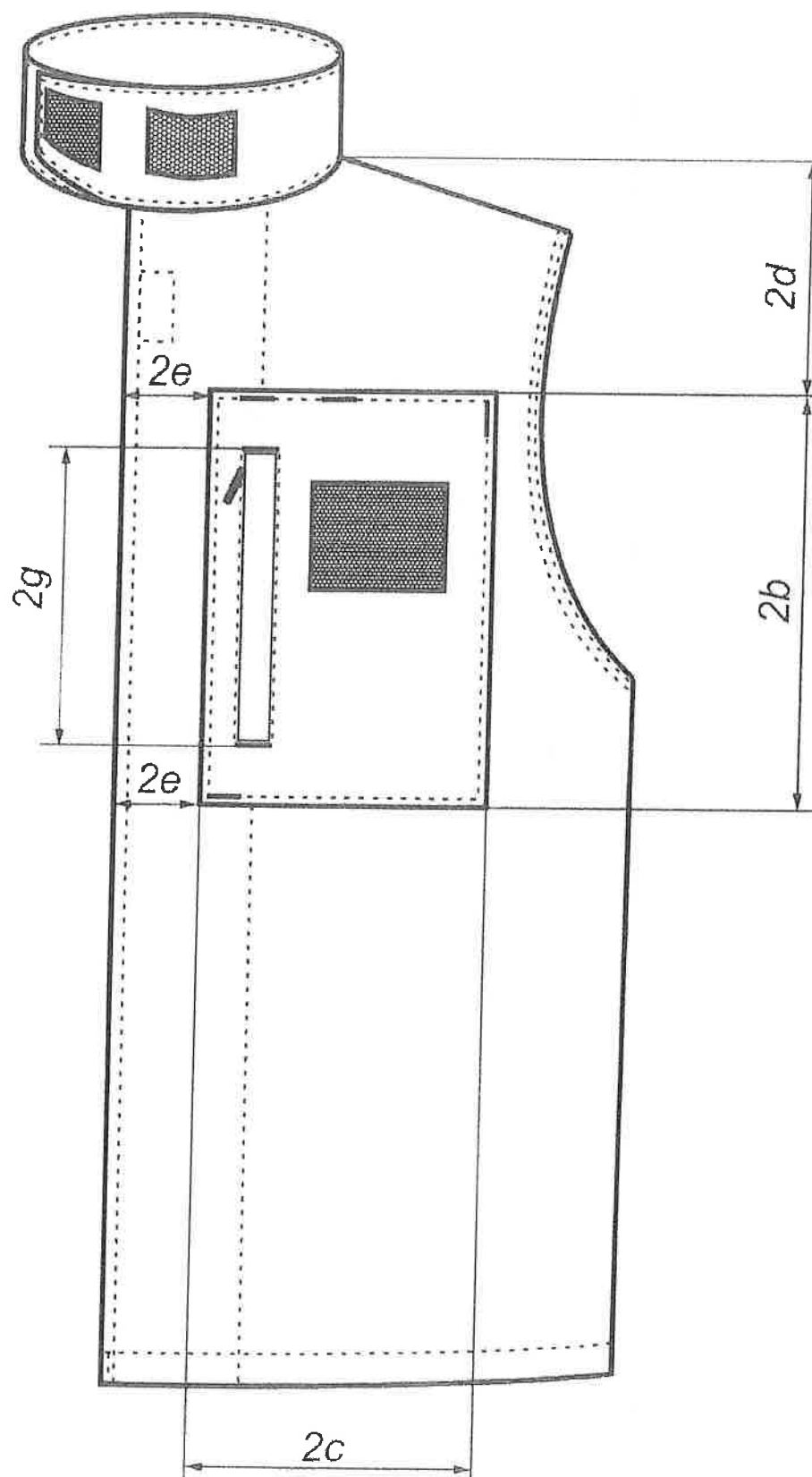
Rysunek 3 – Przód bluzy rozmieszczenie kieszeni
