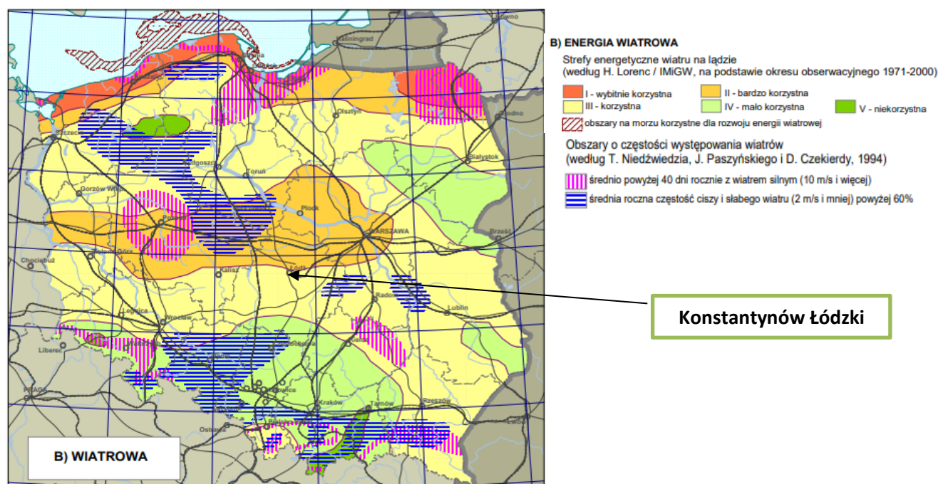
Rysunek 6. Strefy energetyczne wiatru na lądzie (według H. Lorenc/IMI GW, na podstawie okresu obserwacyjnego 1971-2000)
