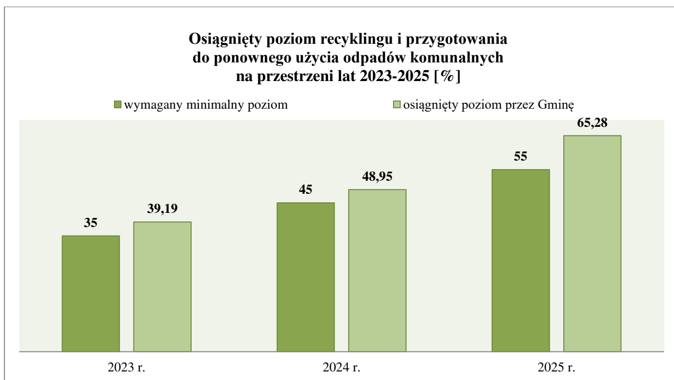
Ryc. 42 Osiągnięty poziom recyklingu i przygotowania do ponownego użycia odpadów komunalnych na przestrzeni lat 2023 - 2025.
