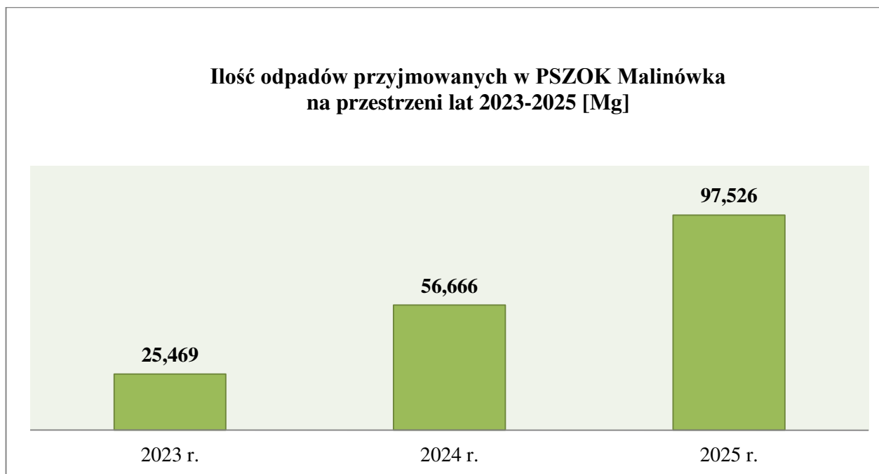
Ryc. 41 Ilość odpadów przyjmowanych w PSZOK Malinówka na przestrzeni lat 2023 - 2025.
