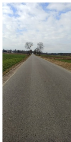
Przebudowa drogi powiatowej nr 2124W Orzyc - Magnuszew Mały - Przeradowo 3,272 km - zadanie rozpoczęte i zakończone w 2021 roku
