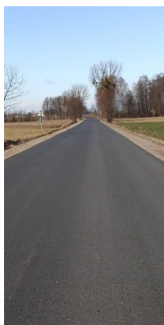
Przebudowa drogi powiatowej nr 2132W Krasnosielc - Pienice - Młynarze 1,800 km – zadanie rozpoczęte w 2021 roku
