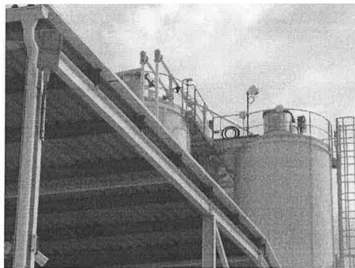
Widok obiektu wraz z zainstalowanym zespołem antenowym
