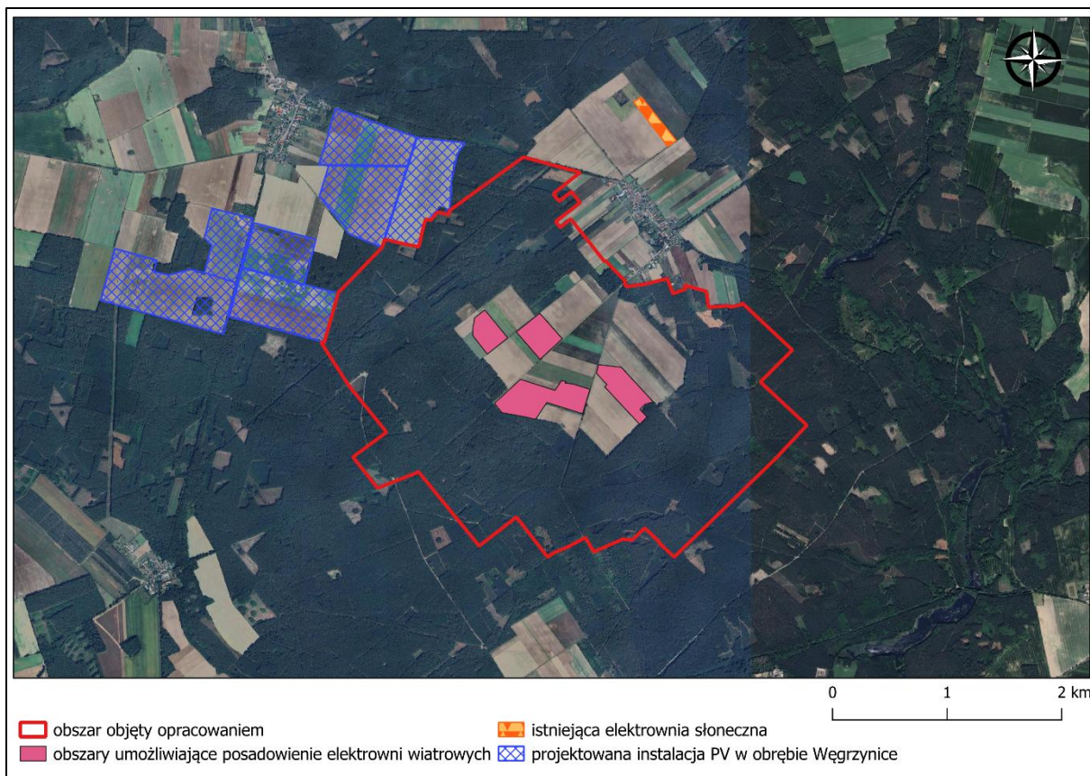
Rysunek 17. Lokalizacja projektu planu i projektowanej elektrowni słonecznej na tle ortofotomapy obrazującej oddzielające inwestycje lasy
