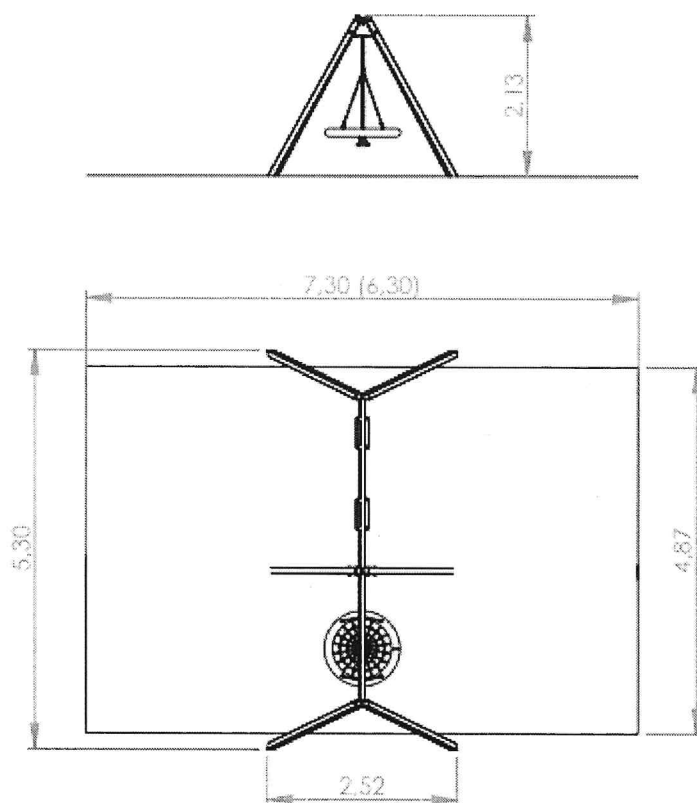
Minimalna strefa użytkowania urządzenia zabawowego
