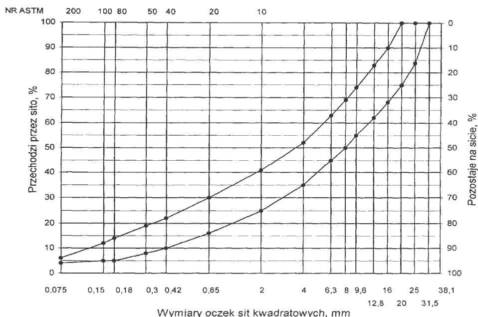
Rys. 2. Krzywe graniczne uziarnienia mieszanek mineralnych BA od 0 do 20 mm do warstwy wiążącej, wyrównawczej i wzmacniającej nawierzchni drogi o obciążeniu ruchem od KR3 do KR6
