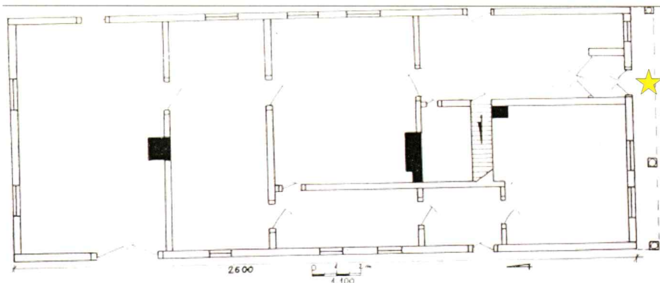
Il. 2. Dom podcieniowy z lokalizacją kolumny przeznaczonej do rekonstrukcji ★ (na podstawie: Karta ewidencyjna, Stary dom – Gminny Ośrodek Kultury, Solec nad Wisłą , oprac. J. Szałygin, 1998).
