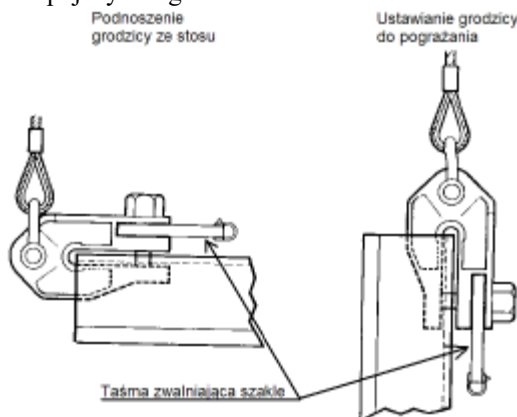
Rysunek 1. Szakla zwalniane z powierzchni terenu
