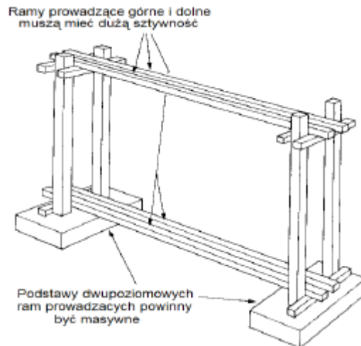
Rysunek 10. Dwupoziomowa rama prowadząca
