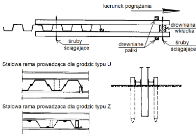
Rysunek 9. Drewniane oraz stalowe ramy prowadzące jednopoziomowe
