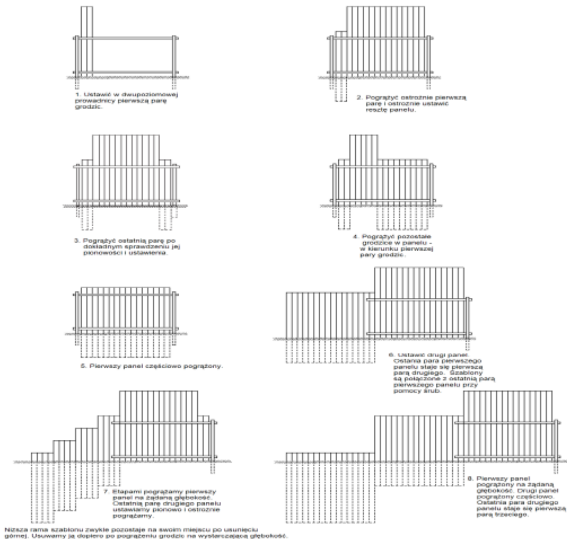
Rysunek 2. Metoda pograżania panelowego.
