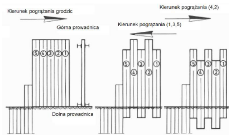
Rysunek 2. Metoda pograżania panelowego.
