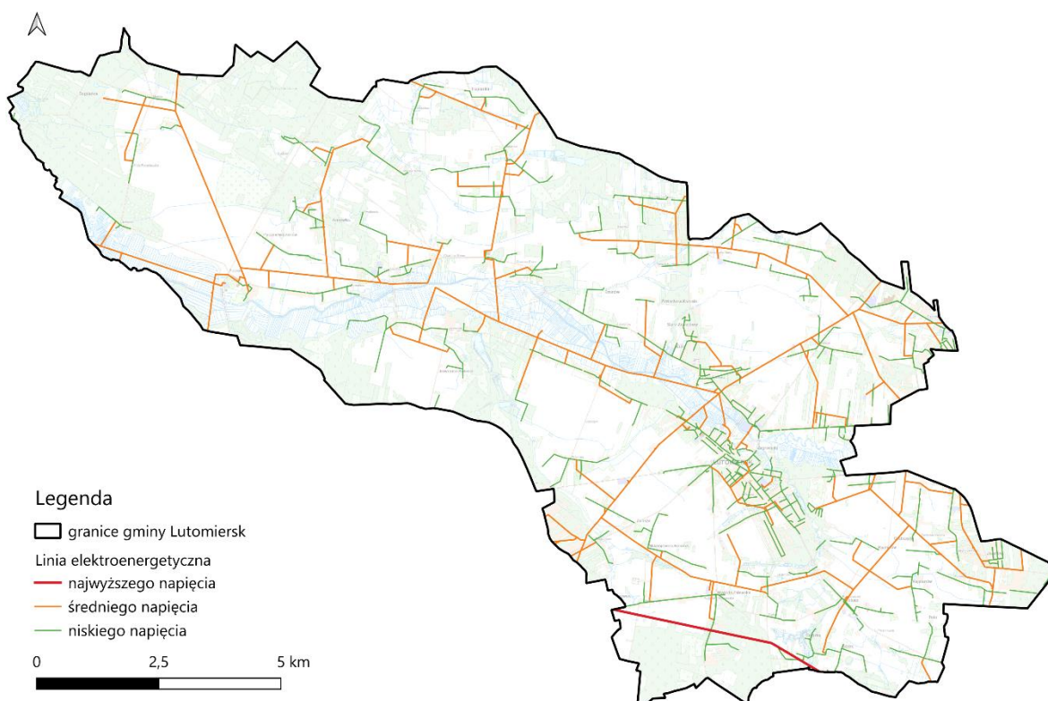
Rysunek 17. Linie elektroenergetyczne na tle gminy Lutomiersk źródło: opracowane własne na podstawie danych geoprzestrzennych
