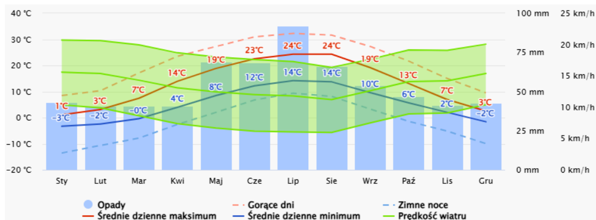
Rysunek 3. Średnie temperatury, opady oraz prędkość wiatru na terenie gminy Lutomiersk źródło: www.meteoblue.com [data dostępu: 18.08.2026 r.]
