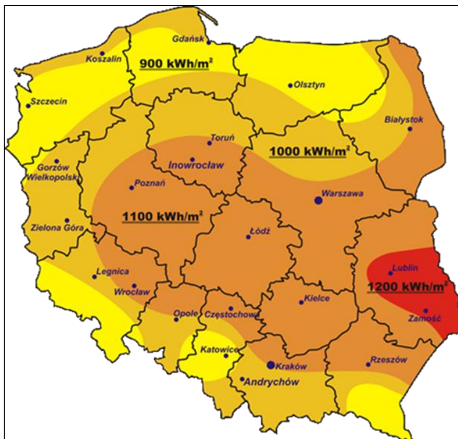
Rysunek 14. Mapa nasłonecznienia Polski źródło: cire.pl
