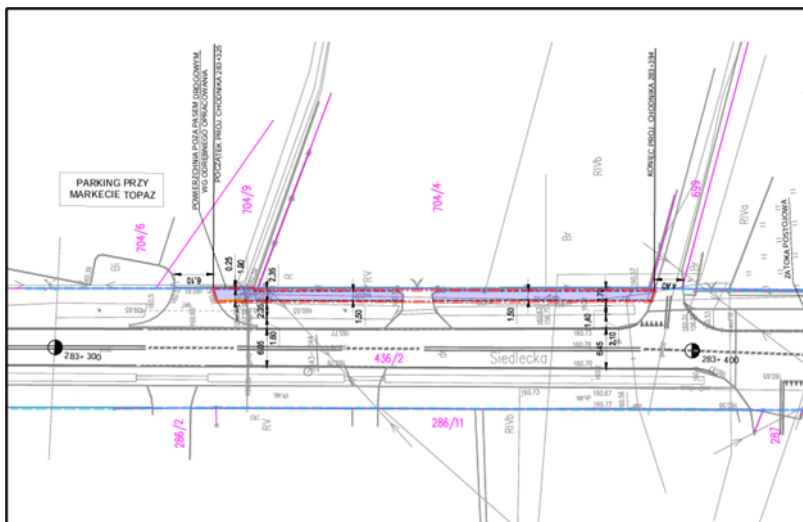
Rycina 11 Mapa budowy chodnika w Wiśniewie
