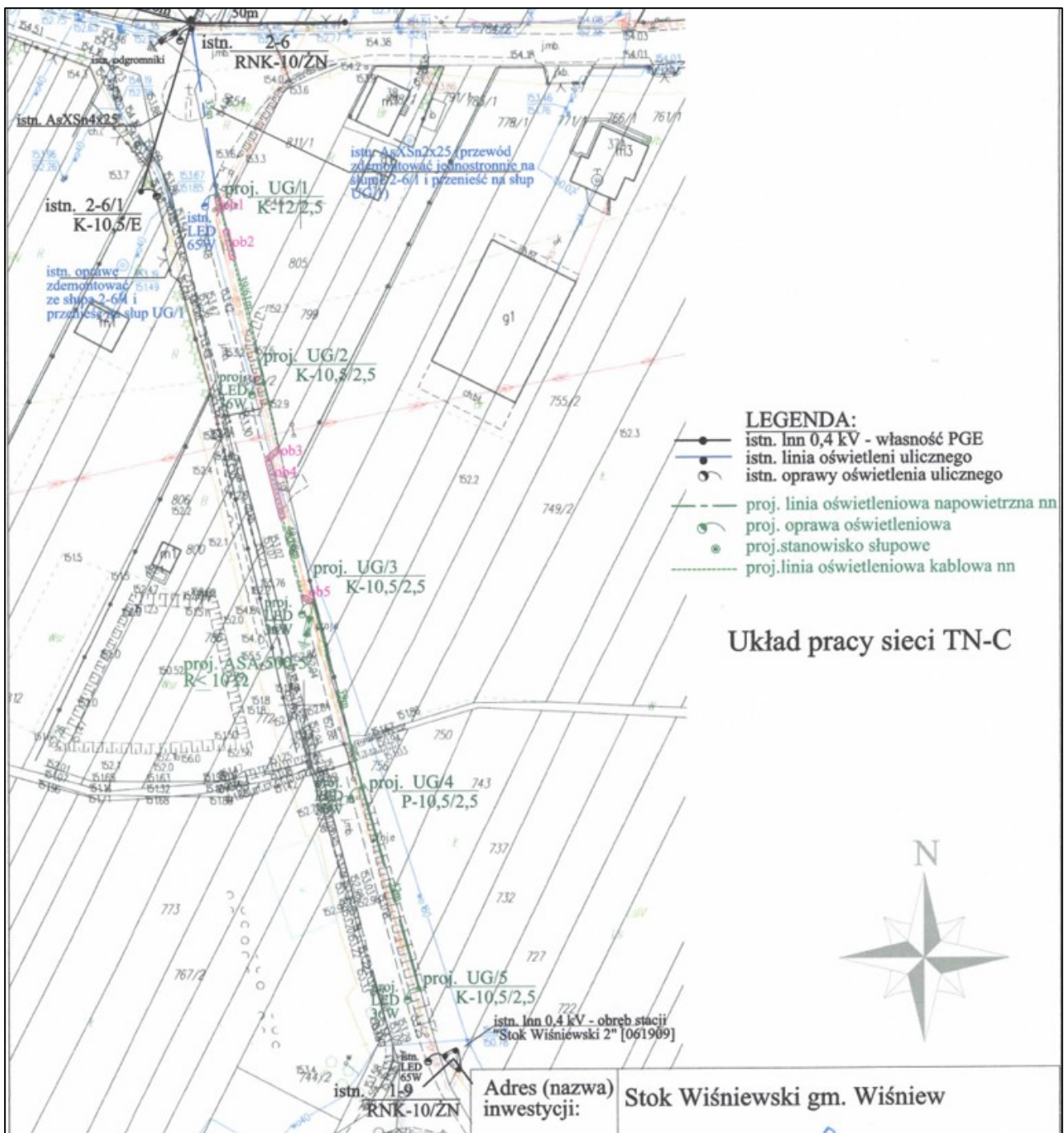
Rycina 5 Projekt oświetlenia ulicznego w miejscowości Stok Wiśniewski
