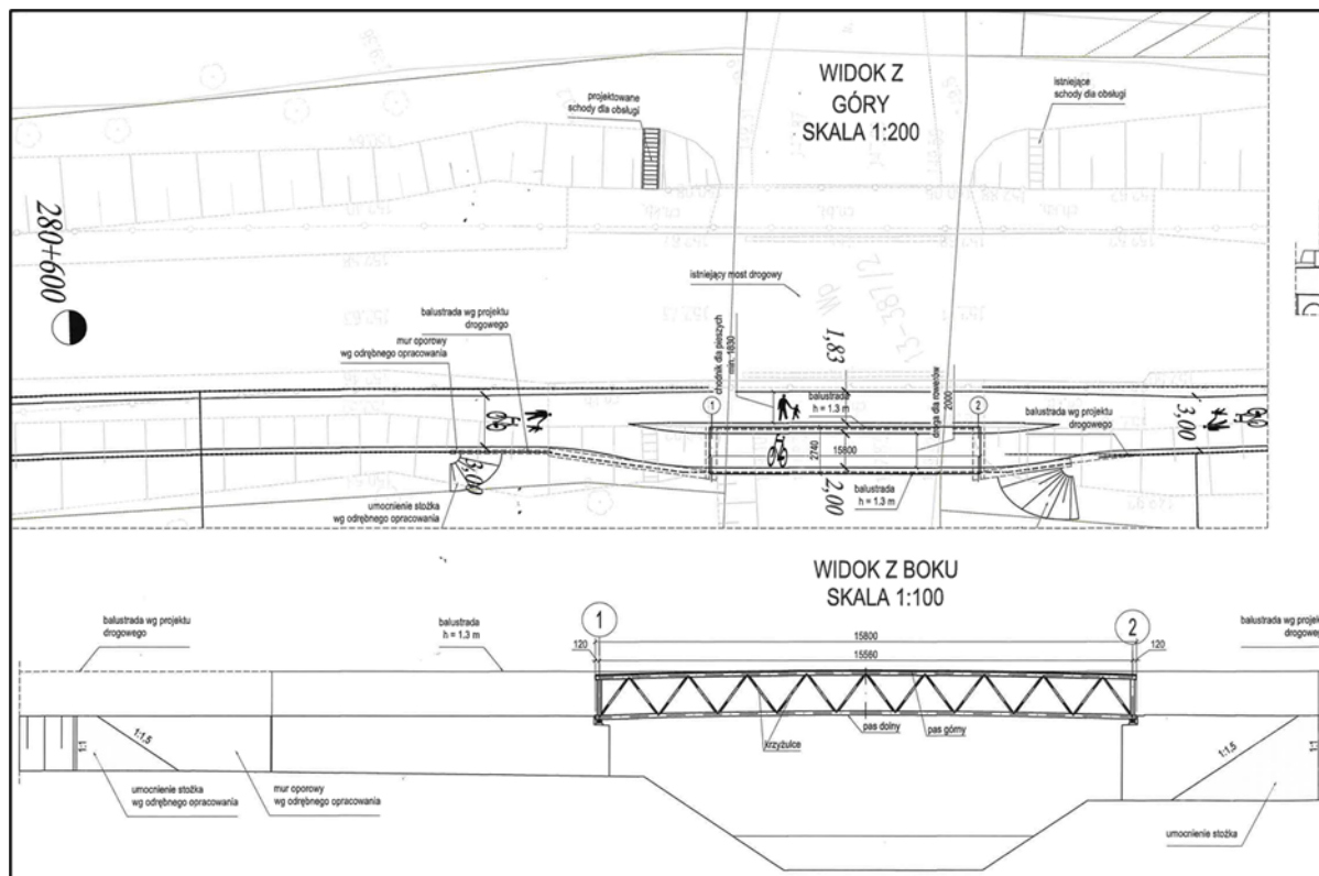
Rycina 2 Plan inwestycji drogi dla rowerów i pieszych
