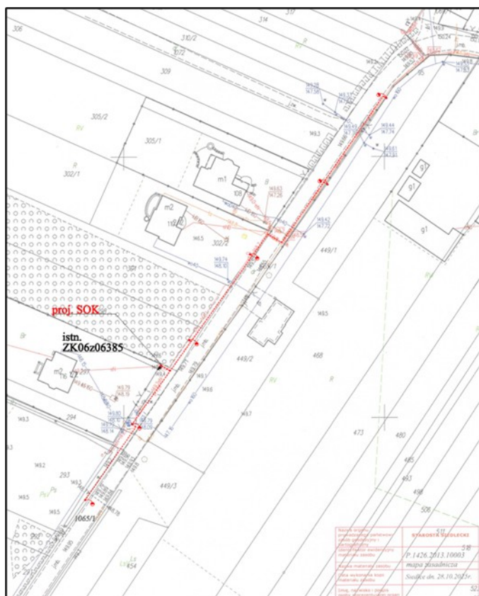
Rycina 9 Projekt oświetlenia ulicznego w Wólce Wiśniewskiej
