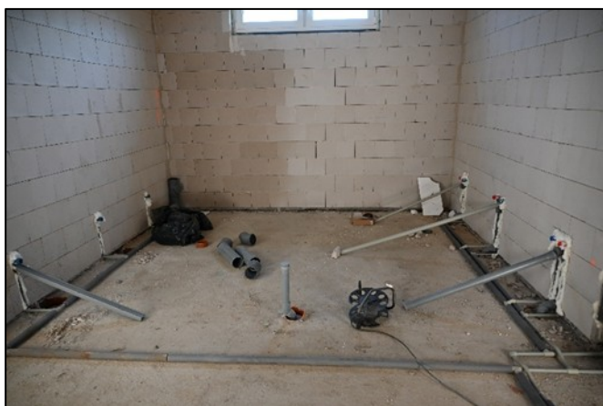
Zdjęcie 25 Budowa żłobka
