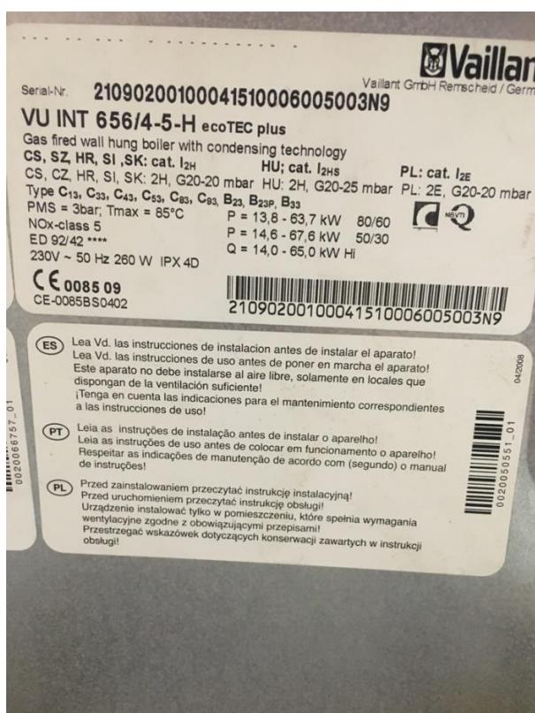
zdj. 3. – tabliczka znamionowa uszkodzonego kotła
