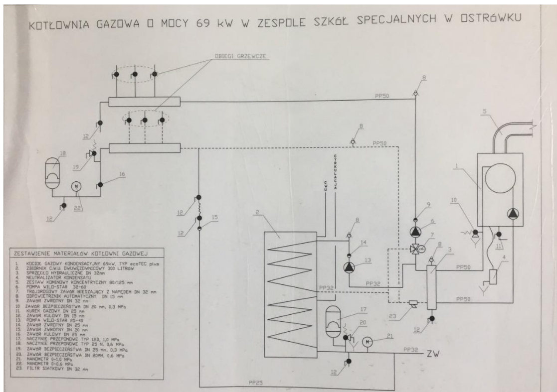
zdj. 2 – schemat kotłowni
