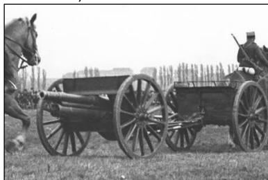
Fot. Armata polowa 85mm z zaprzęgiem
