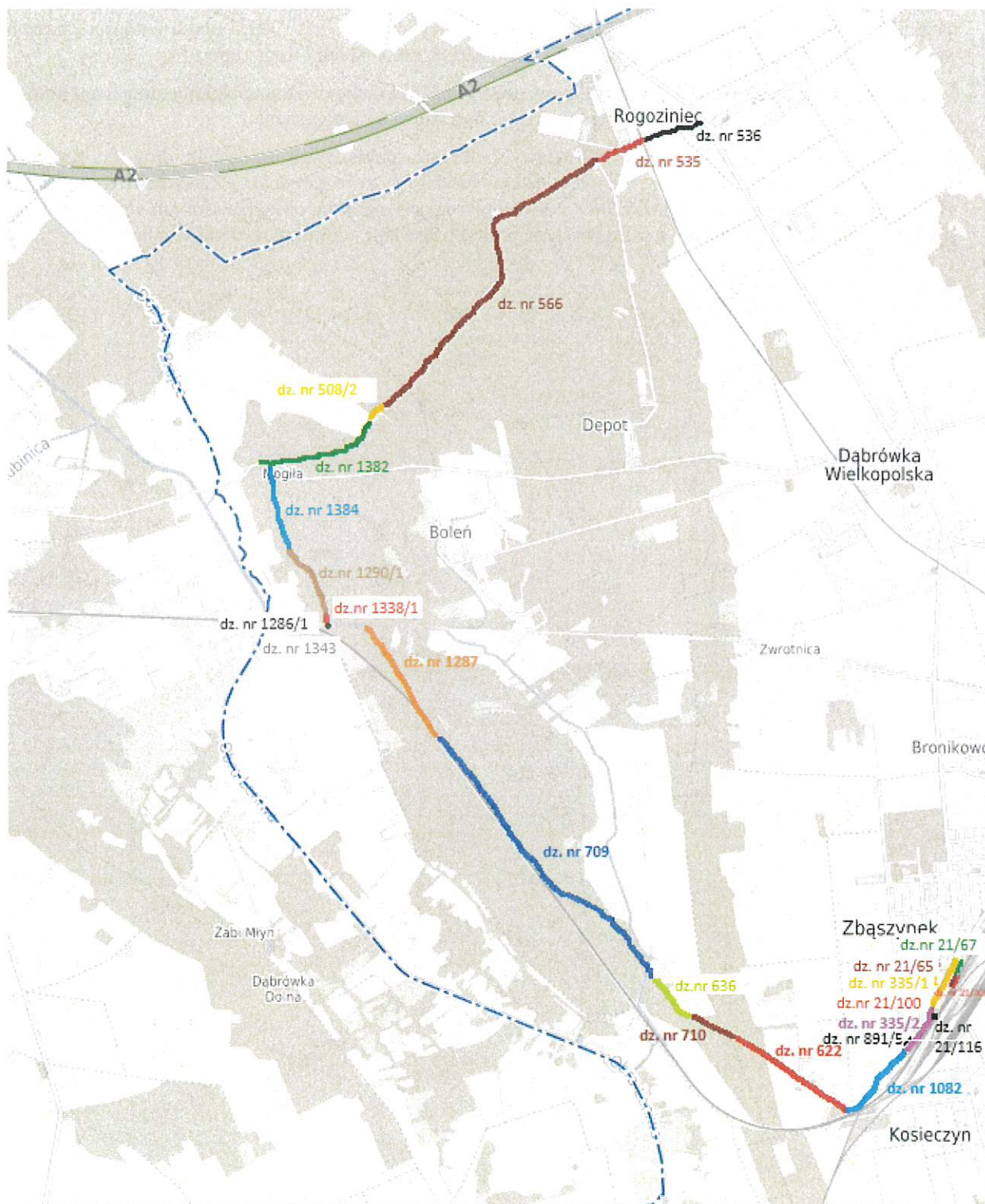
Nowy przebieg drogi powiatowej nr 1212F relacji Zbąszynek- Boleń – Rogoziniec.
